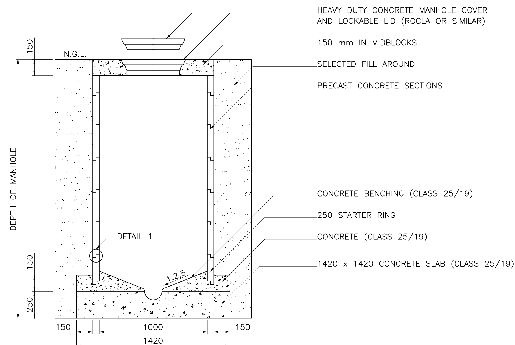
SECTION A-A
