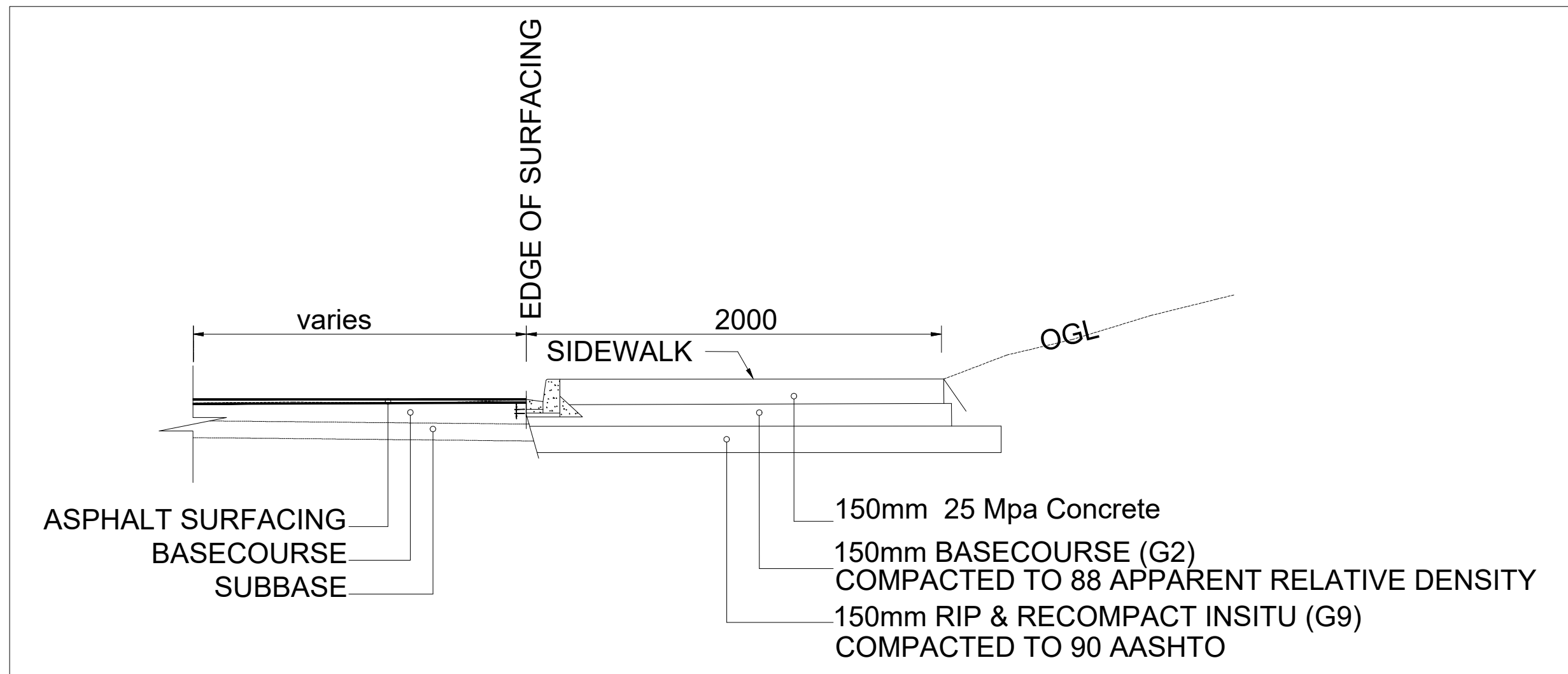
SIDEWALK CROSS SECTION N.T.S
