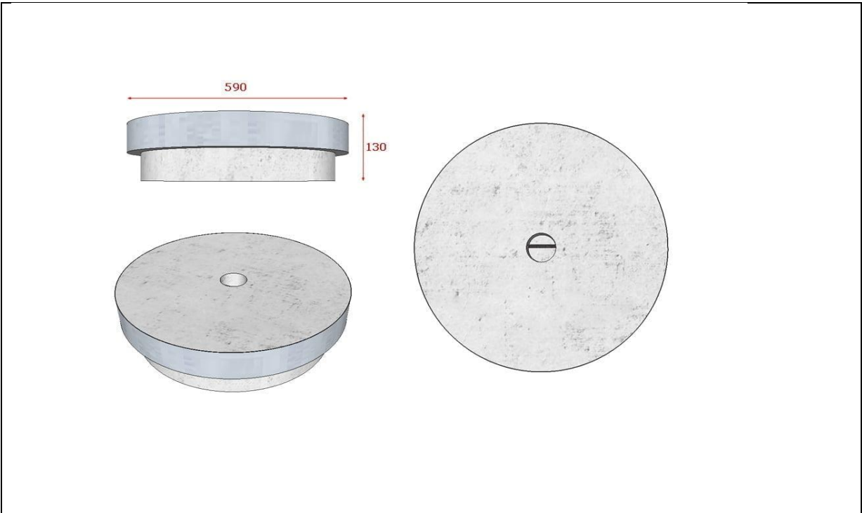
Concrete Lid
