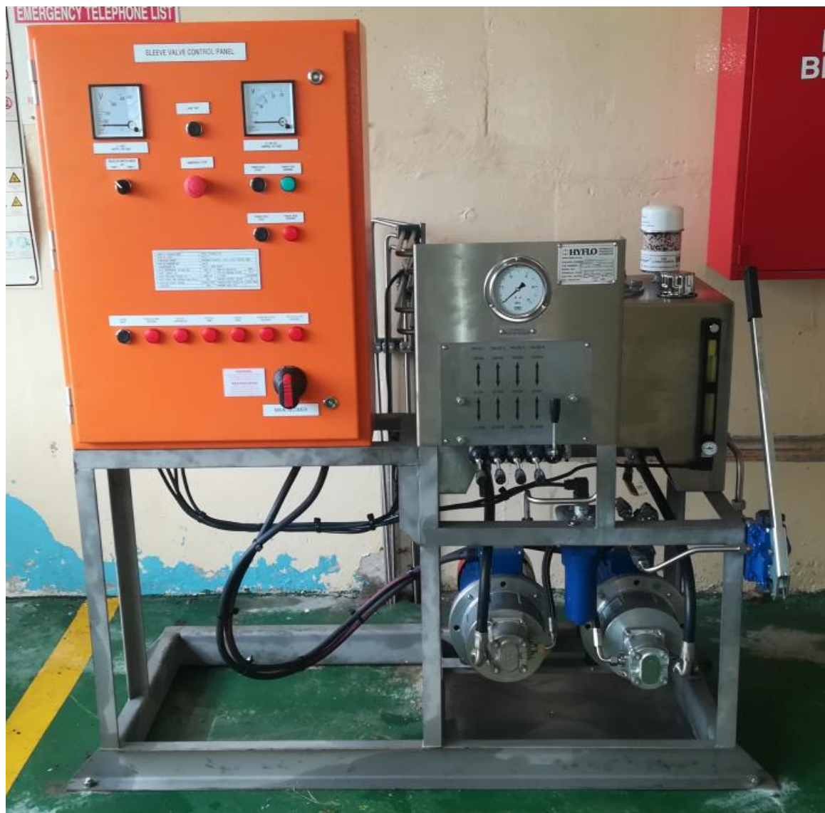
Spioenkop dam: Outlet control room: Hydraulic power pack
