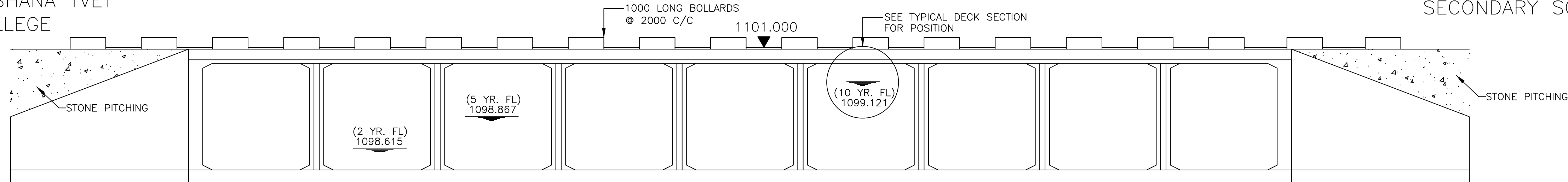
LONGITUDINAL ELEVATION SCALE 1 : 75
