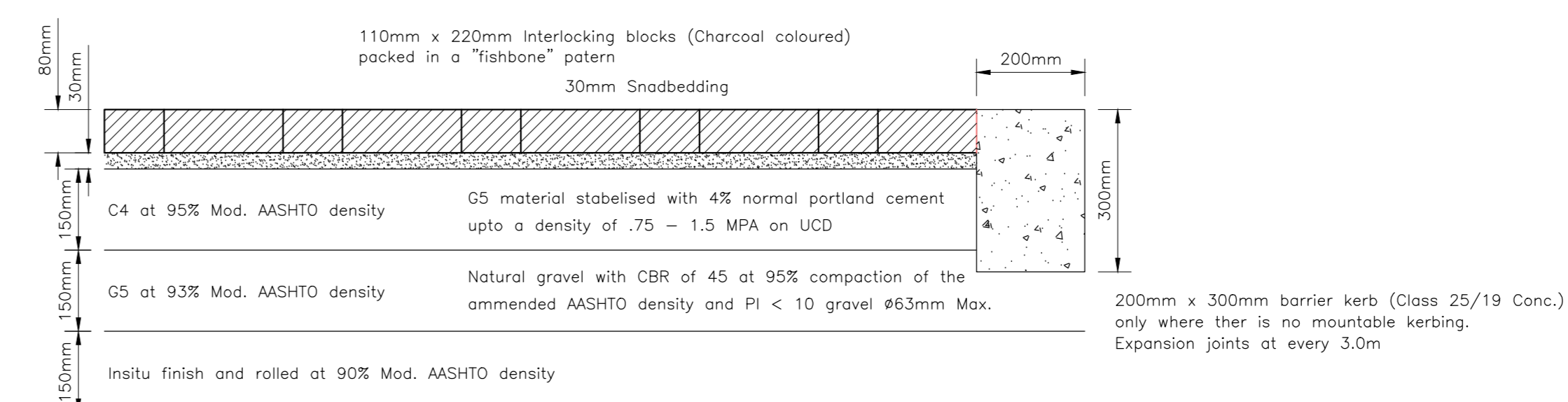
LAYER WORK DETAIL N.T.S.
