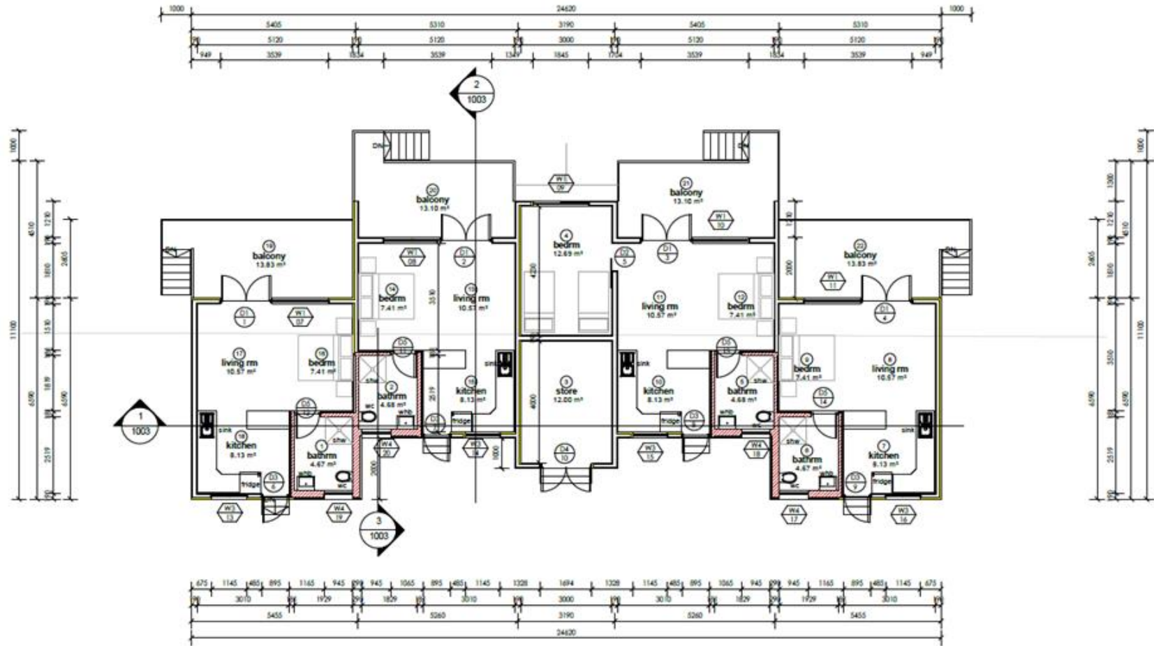
00-Ground Storey Plan Scale: 1 : 100
