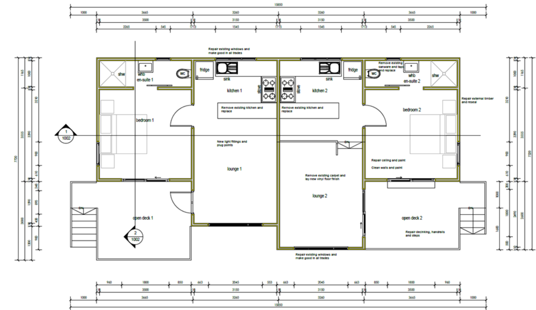
100-Ground Storey Plan Scale: 1 : 50
