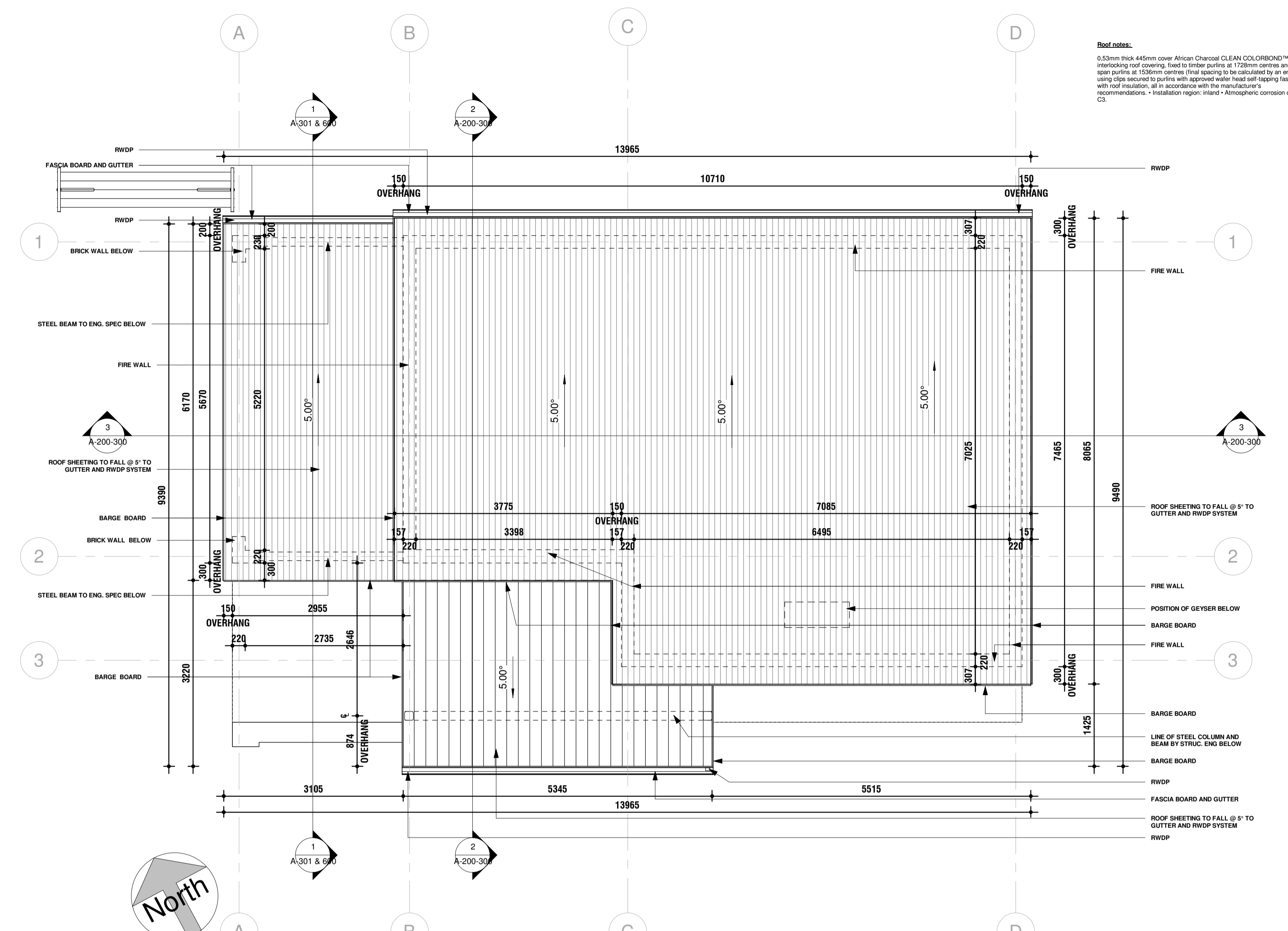
2 Roof plan 1 : 50
