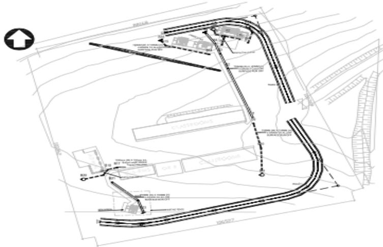
SITE PLAN 1:500
