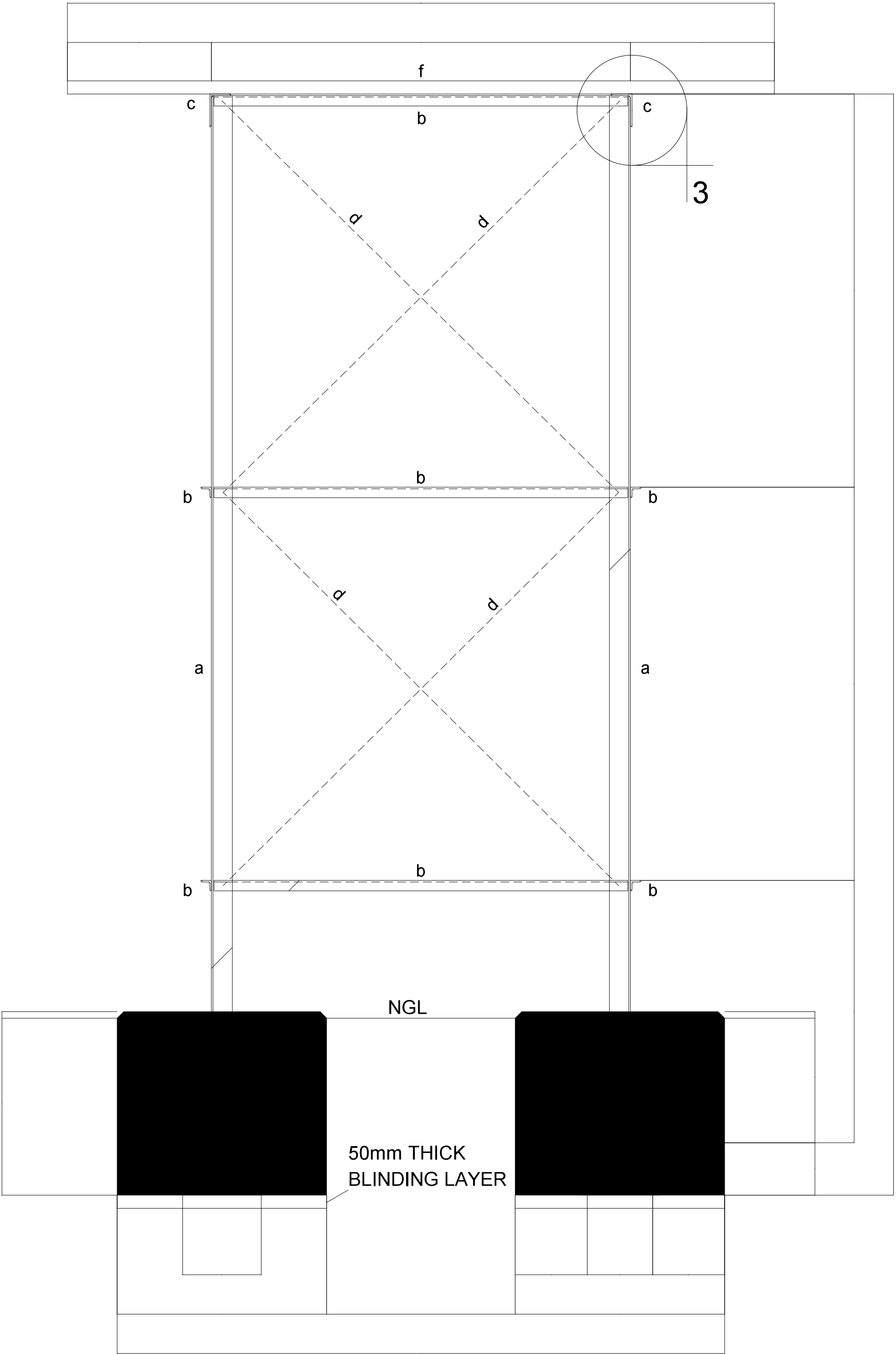
SECTION D-D
