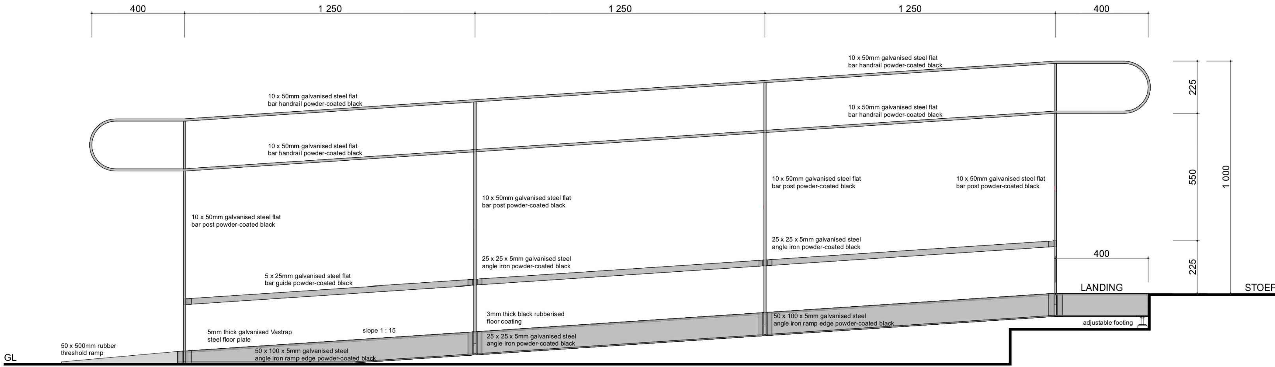
RAMP 2 ELEVATION 1 : 10
