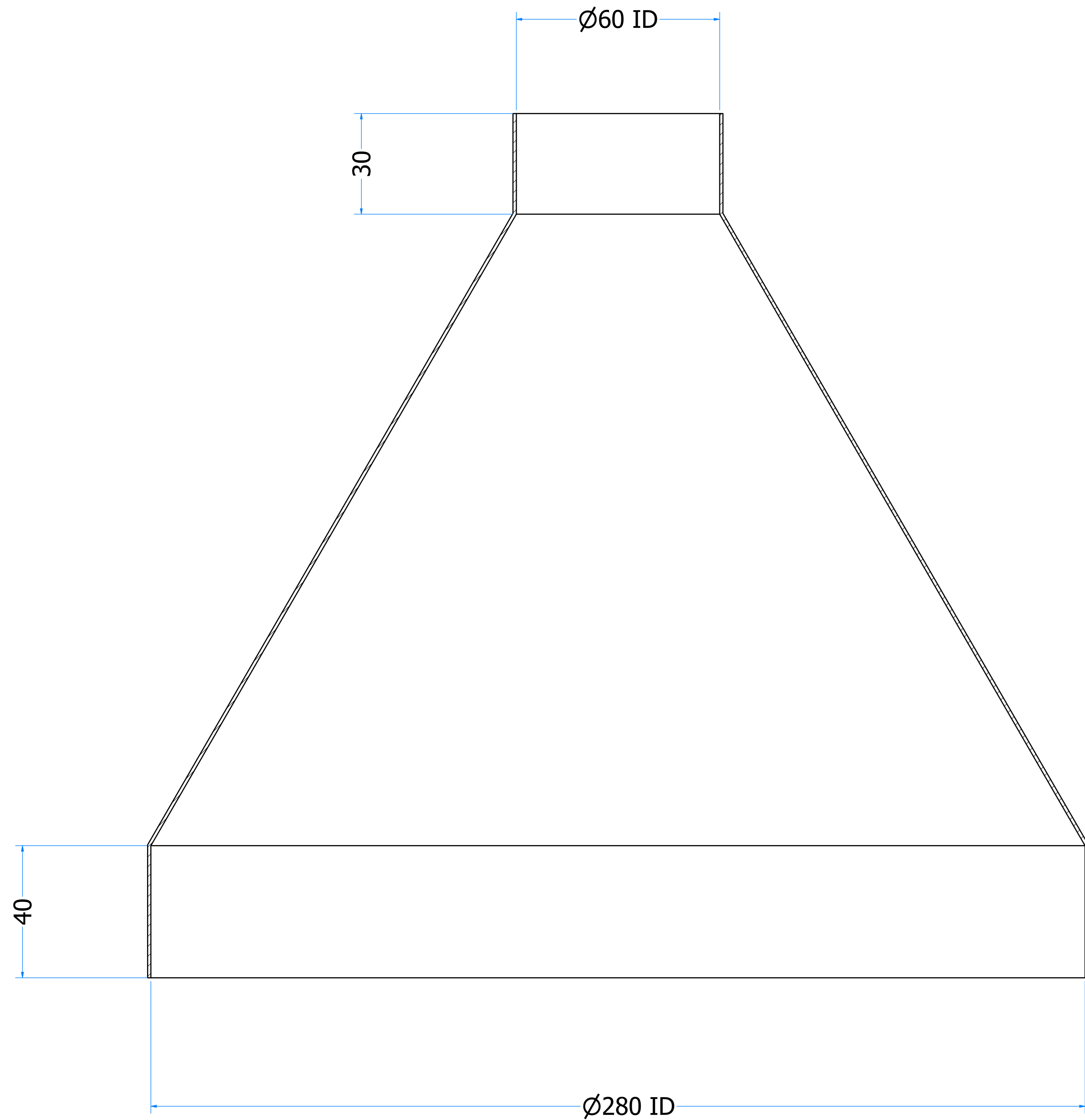
SECTION A-A SCALE 1.5 : 1
