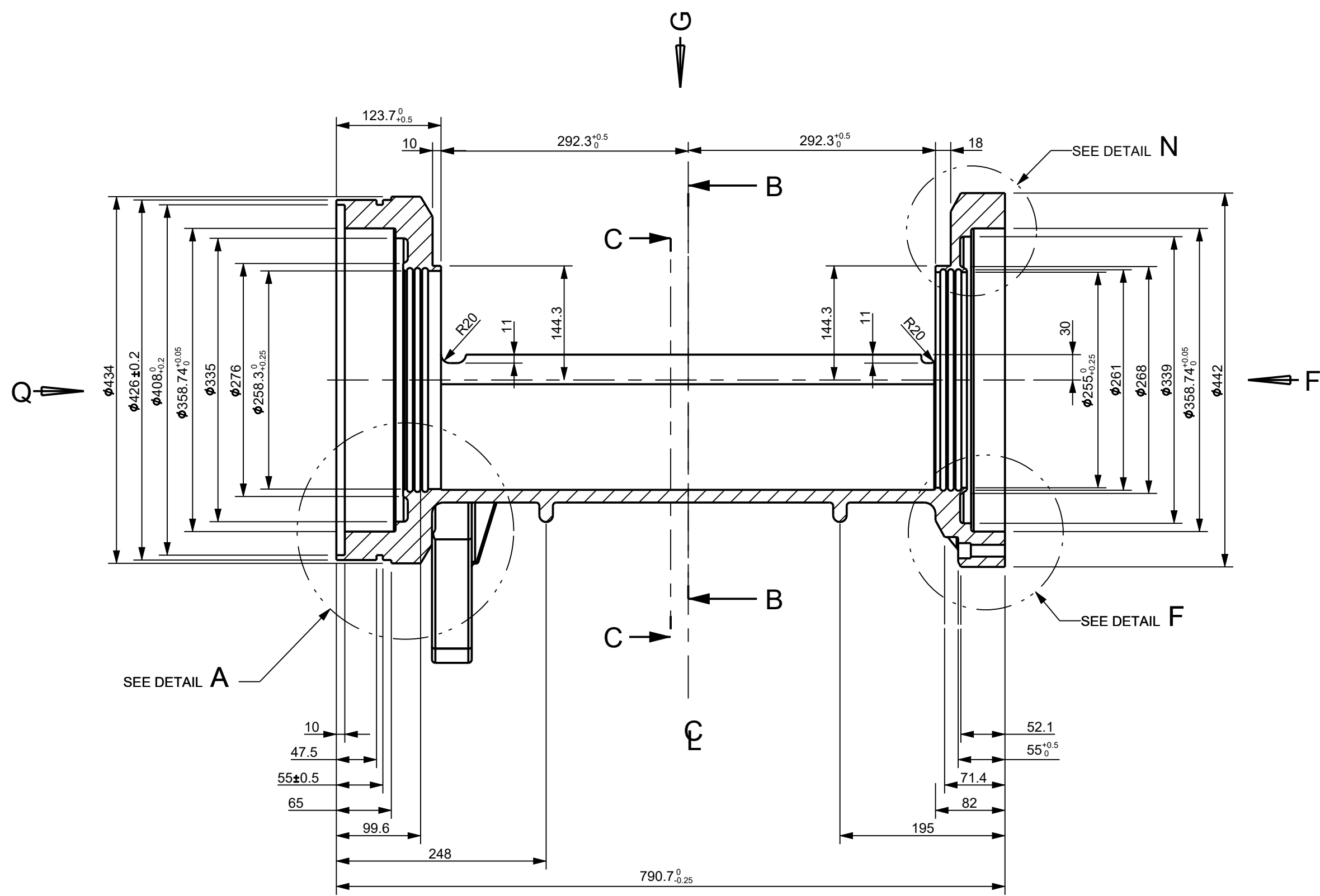
SECTION A-A
