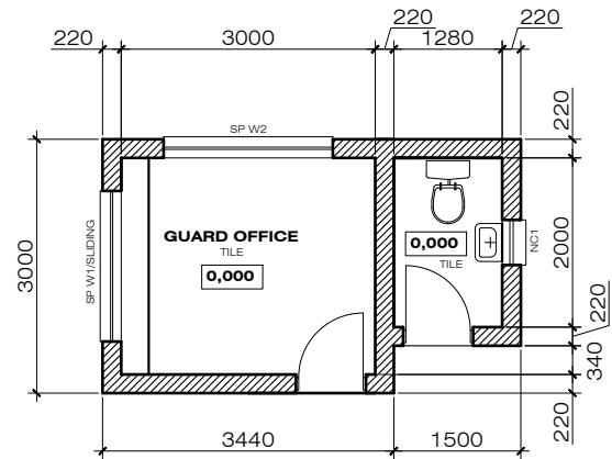
PLAN 1:100
