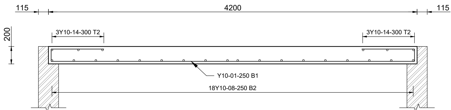
SECTION A-A SCALE 1:25
