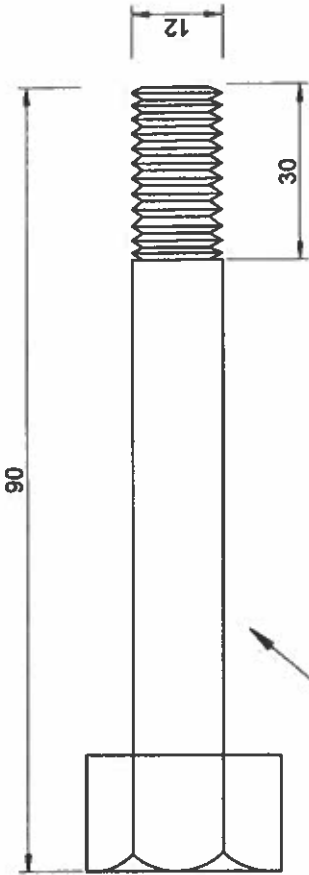
BOLT 1
