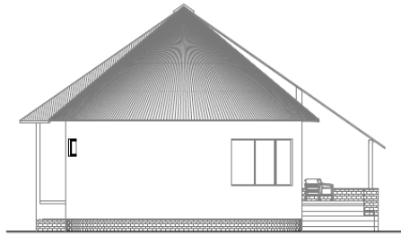
1 Side Elevation Scale: 1 : 100
