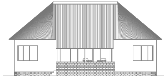
2 Front Elevation Scale: 1 : 100
