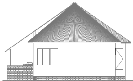
4 Side Elevation Scale: 1 : 100
