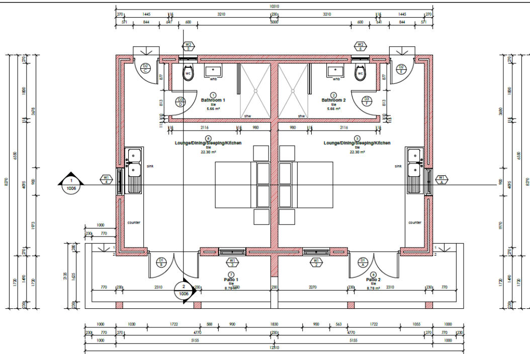
00-Ground Storey Plan Scale: 1 : 50
