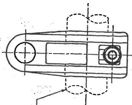
TUBULAR CANTILEVER ARM BUISVORMIGE-VRYDRAERARM
