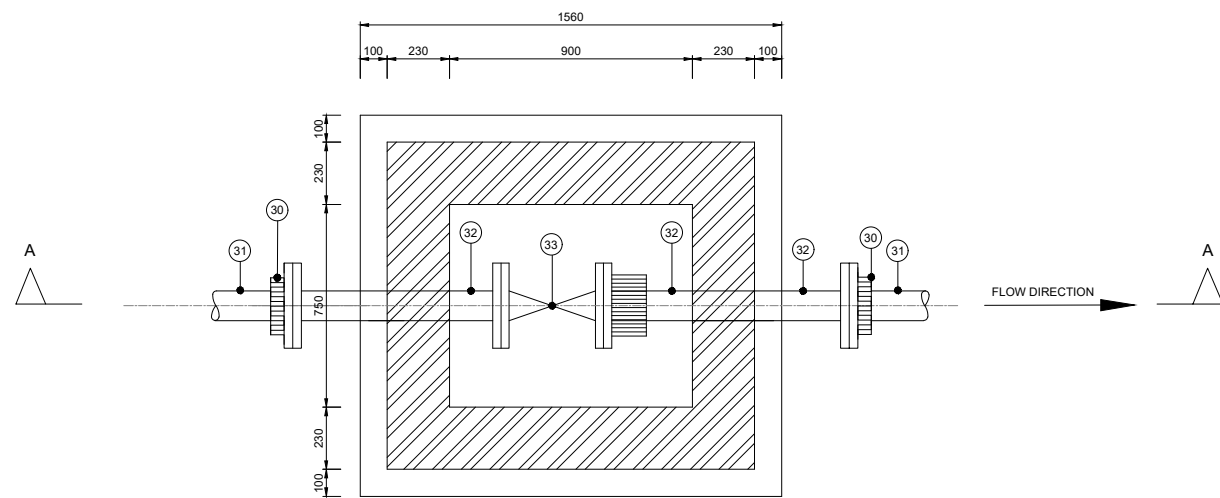
PLAN SCALE: 12.5
