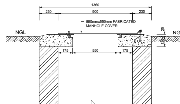
SECTION B-B SCALE: 12.5
