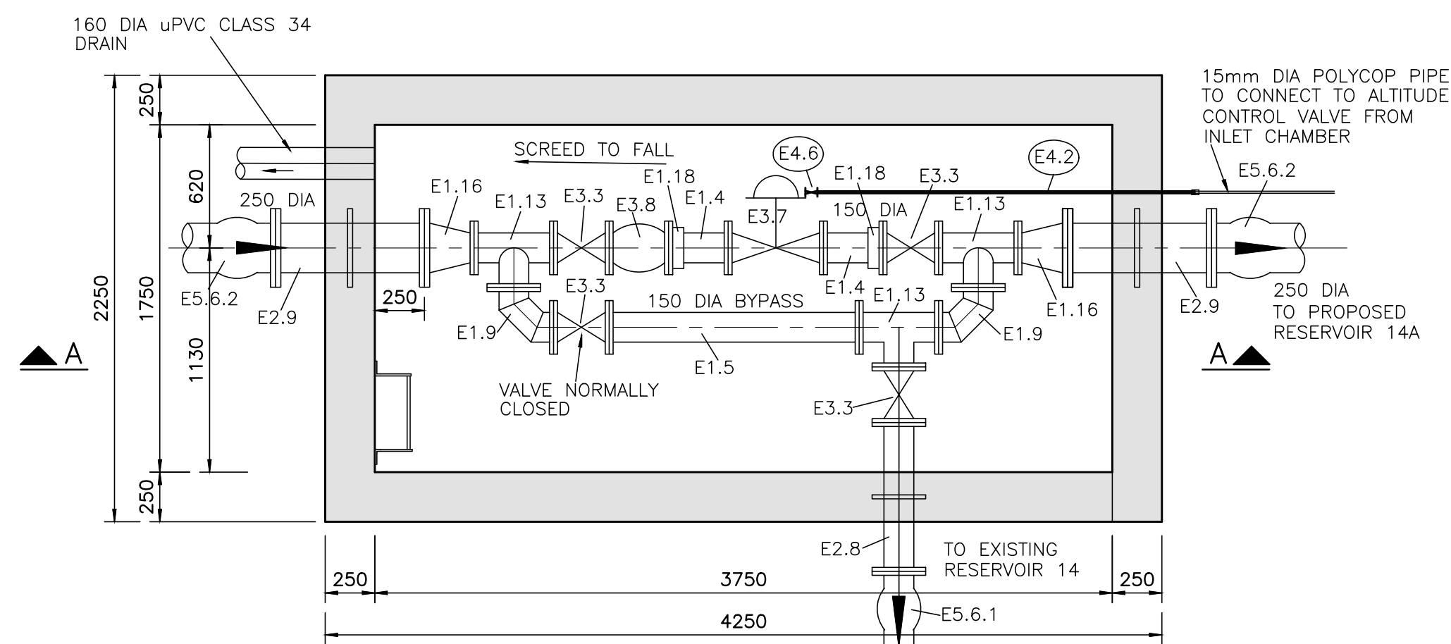
FLOOR PLAN 1 : 25
