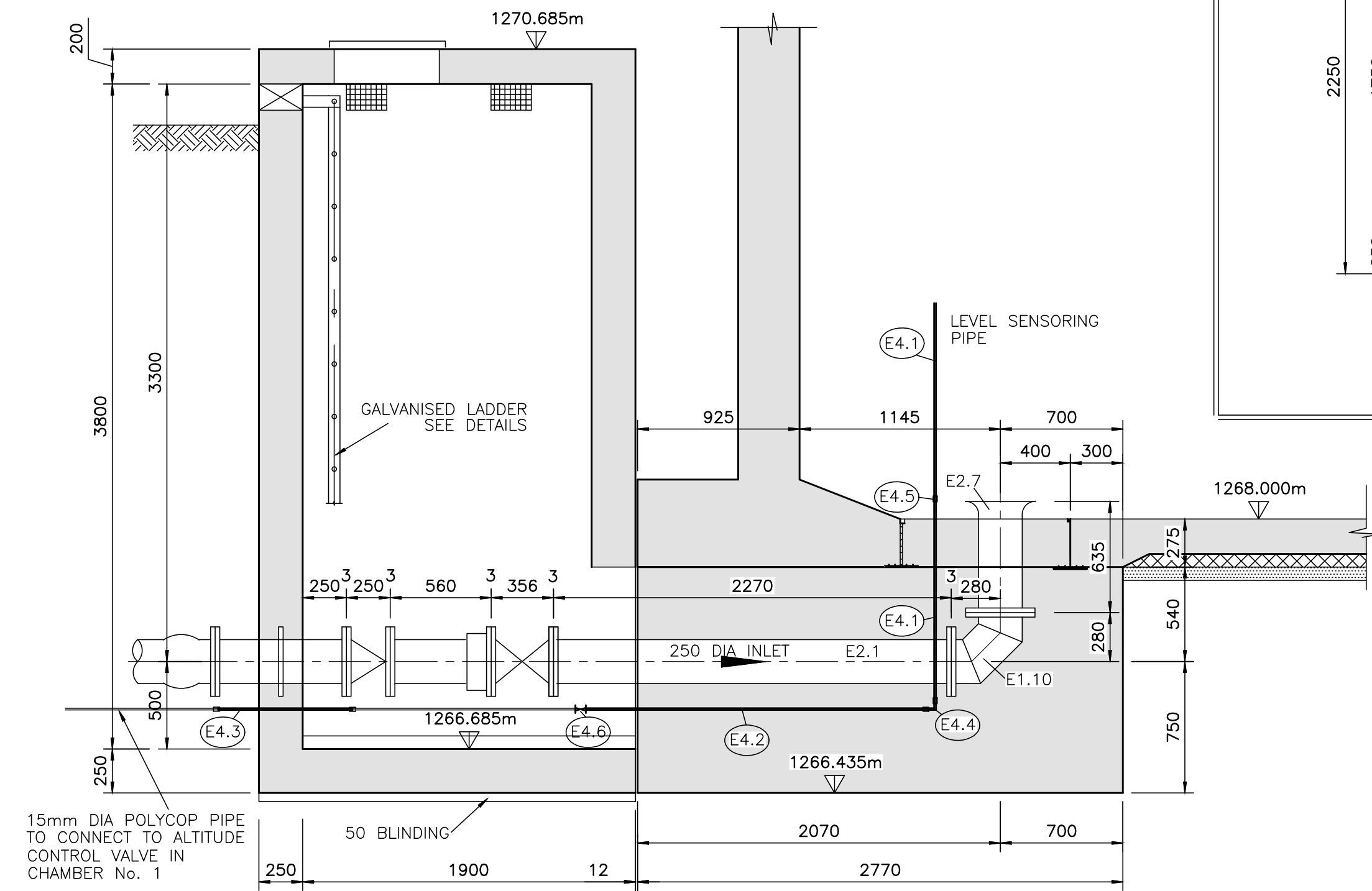
SECTION B - B 1 : 25
