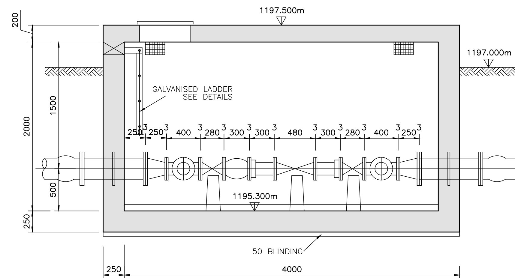
SECTION A - A 1 : 25
