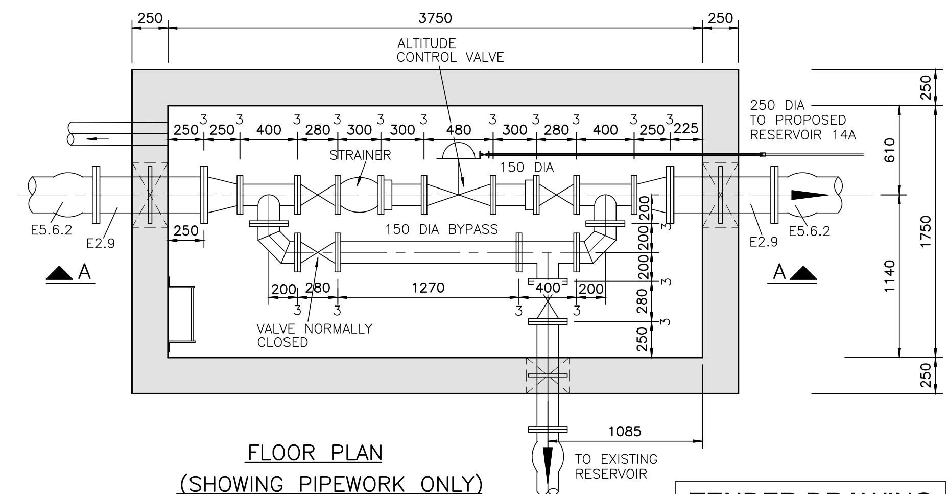
FLOOR PLAN 1 : 25
