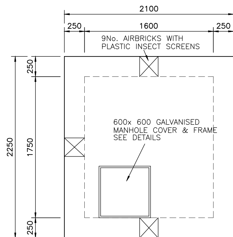
ROOF PLAN 1 : 25
