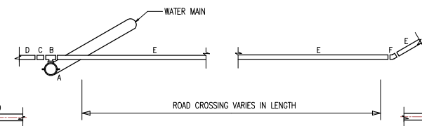
ERF CONNECTION TYPE 8
