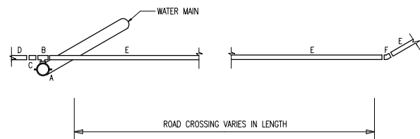
ERF CONNECTION TYPE 5
