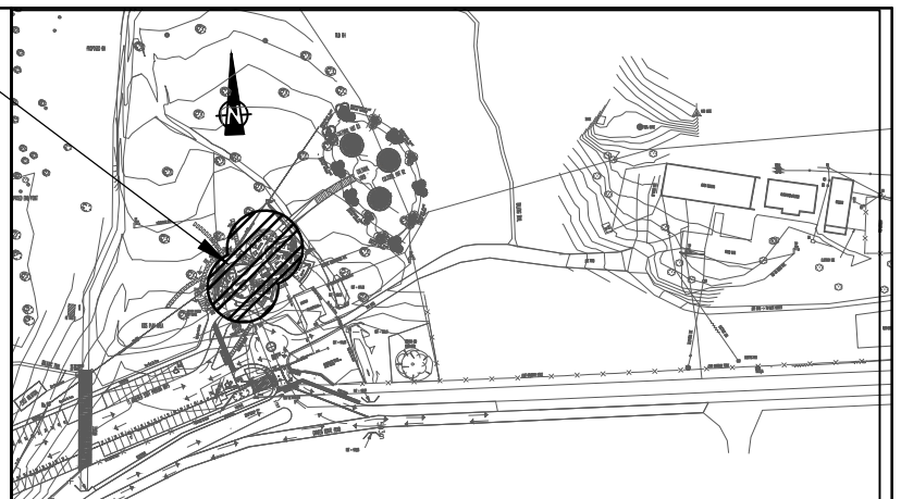
SITE PLAN N.T.S
