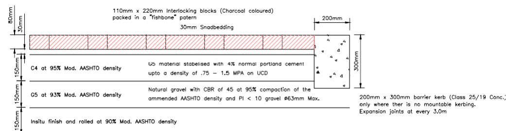
LAYER WORK DETAIL N.T.S.
