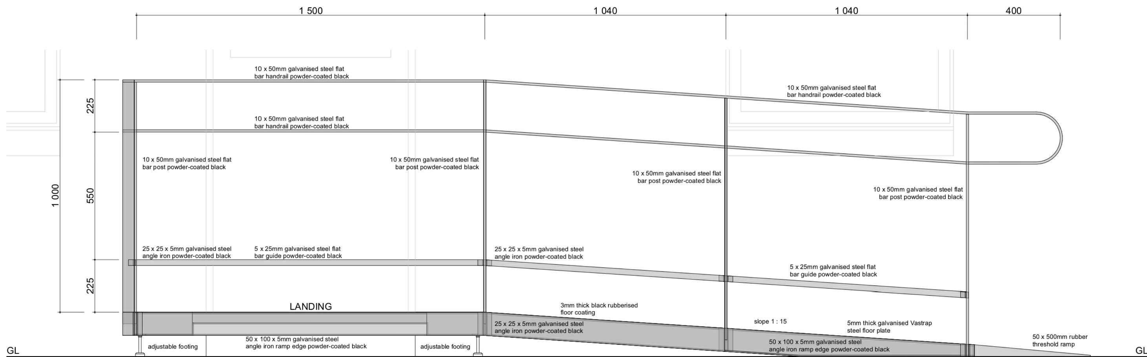
RAMP 3 ELEVATION 1 : 10
