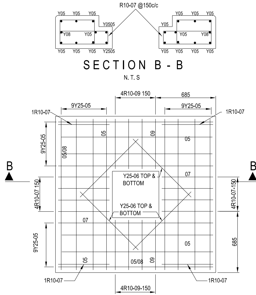
PLAN - REBAR LAYOUT N.T.S
