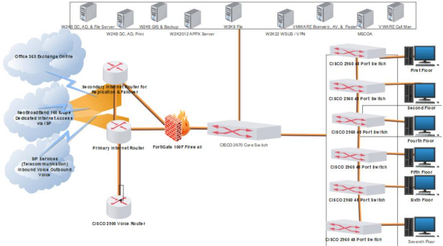
SBDM Local Area Network (LAN) Diagram A:
