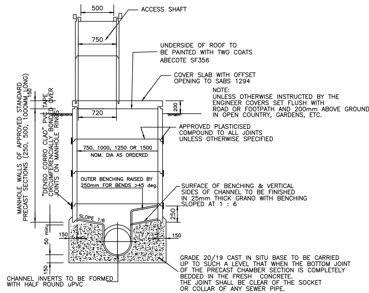
SECTION A-A
