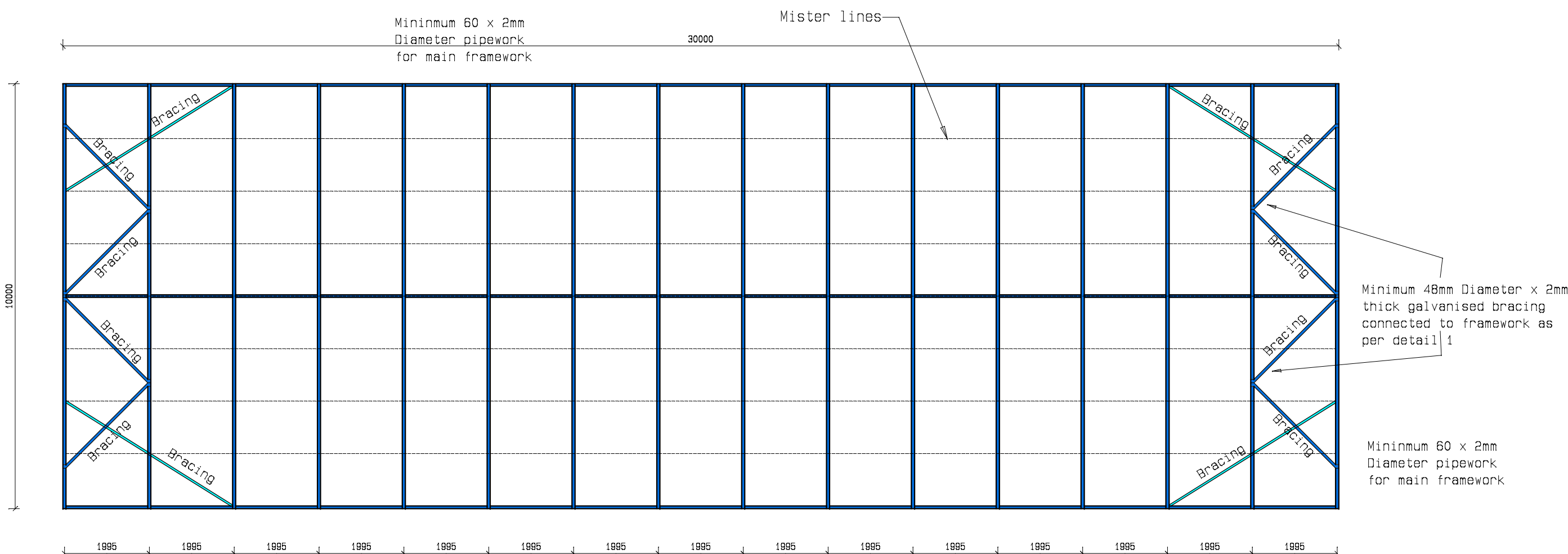
PLAN Scale: 1:100
