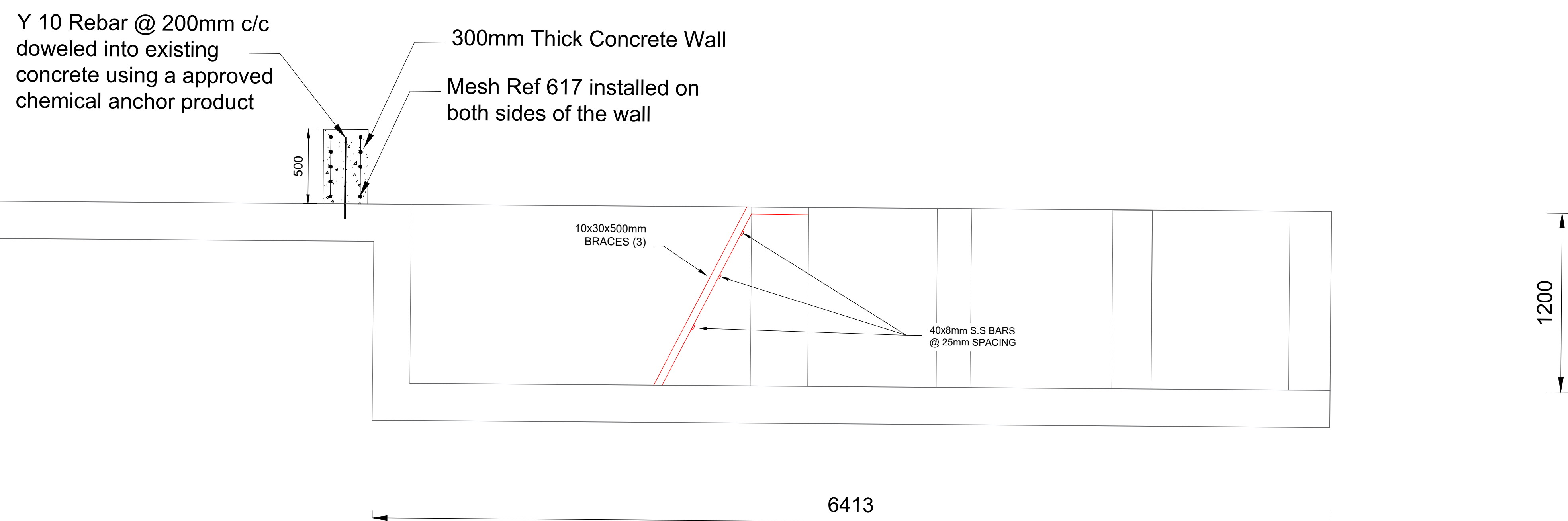
SECTION SCALE 1 : 20
