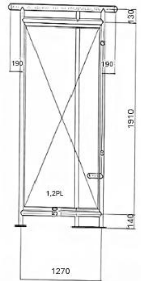
RIGHT ELEV
