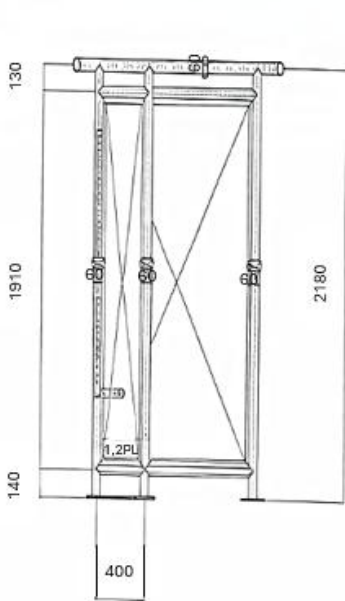
LEFT ELEV
